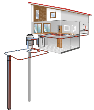
Wärmequelle Erdsonden
